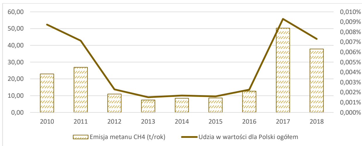
Wykres 8. Emisja metanu CH 4 w latach 2010-2018 (tony)
