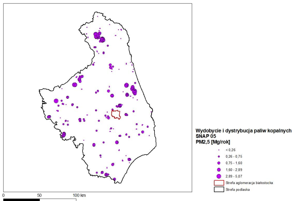
Rysunek 1-68 Rozmieszczenie oraz ładunki emisji punktowej pyłu zawieszonego PM 2,5 w procesie wydobycia i dystrybucji paliw kopalnych (SNAP 05) w strefie podlaskiej w 2018 r.
