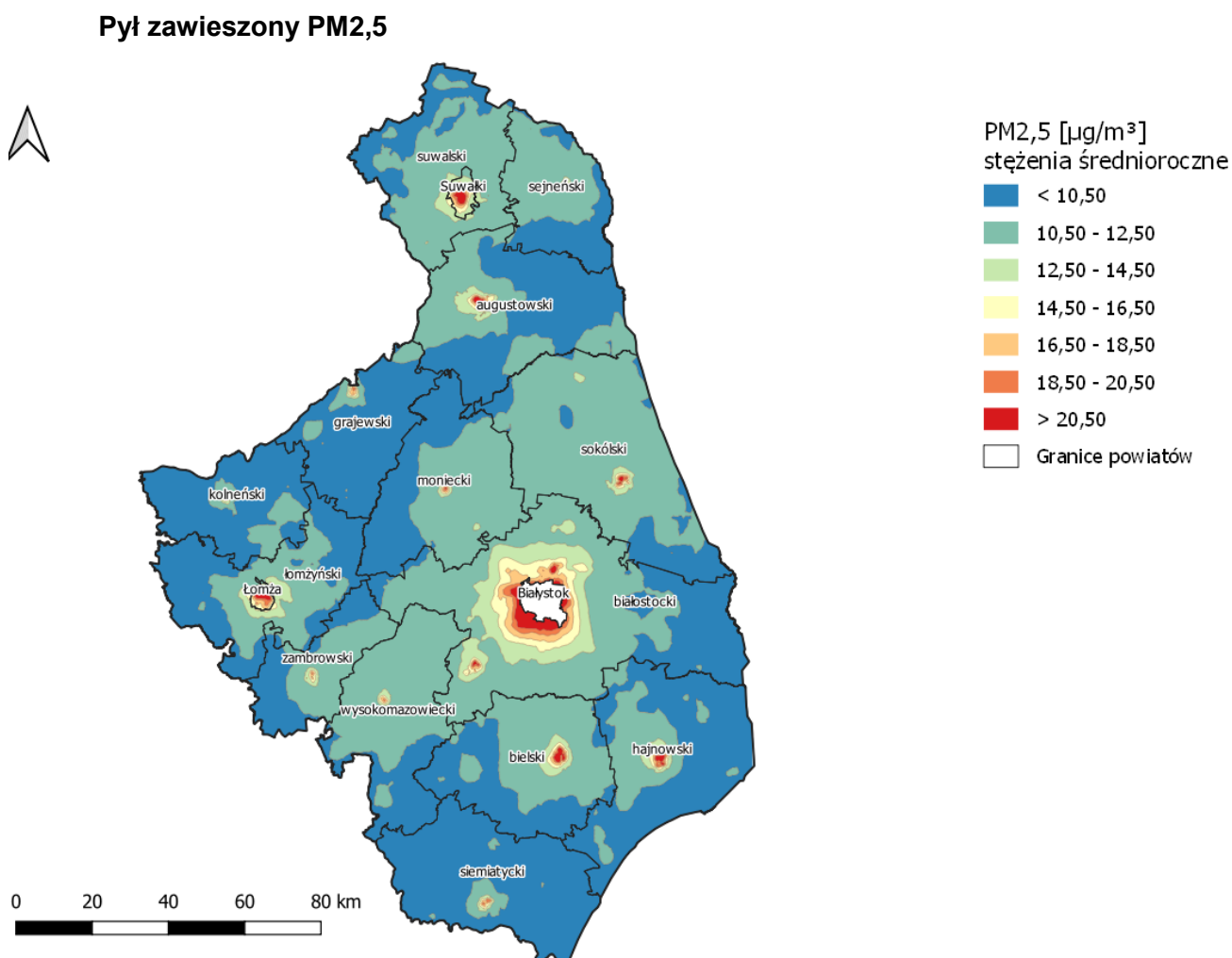
Rysunek 3-2 Rozkłady średniorocznych stężeń pyłu zawieszonego PM 2,5 , w strefie podlaskiej, w 2018 r., dla emisji łącznej wszystkich typów
