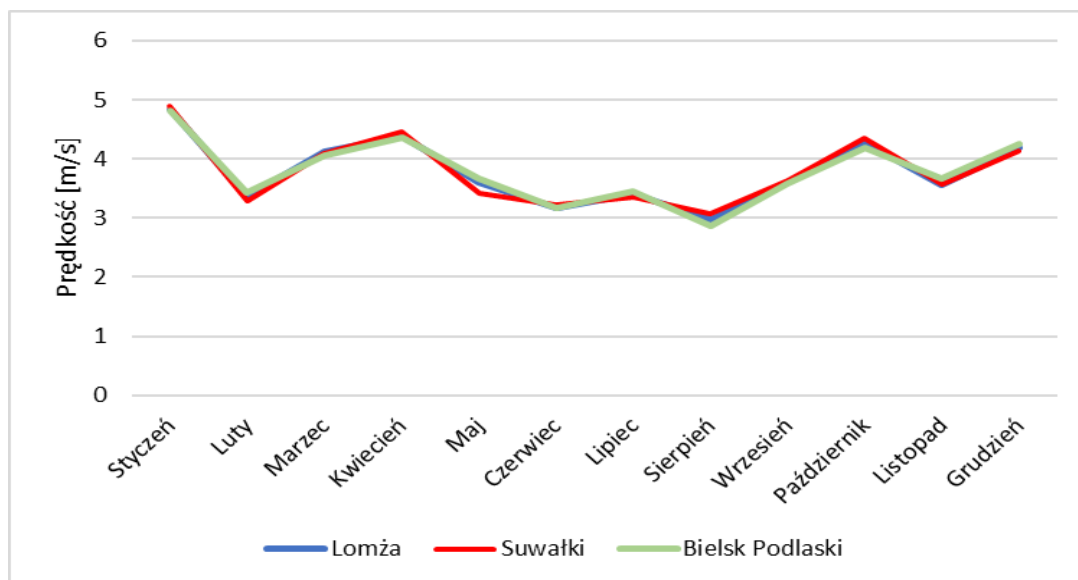
Rysunek 1-8 Średnie miesięczne prędkości wiatru [m/s] wyznaczone przez model WRF/CALMET dla wybranych miejscowości w strefie podlaskiej w 2018 r.
